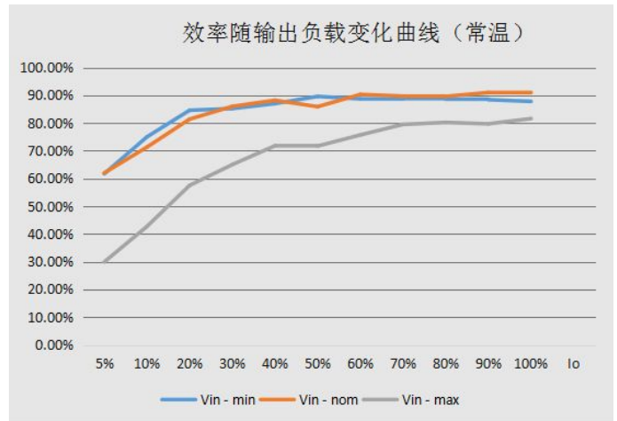
WLD20-H1D54 效率随输出负载变化曲线 (常温)
