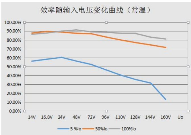
WLD20-H1D54 效率随输入电压变化曲线 (常温)
