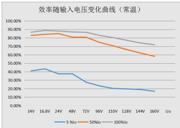
WLD10-H1D54(F/H)效率随输入电压变化曲线 (常温)
