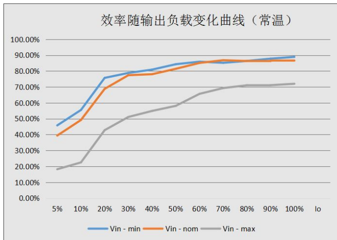
WLD10-H1D54(F/H)效率随输出负载变化曲线 (常温)
