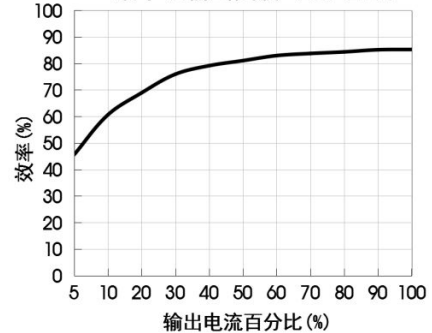
VSD3-B2415 效率Vs输出负载 (Vin=24V)
