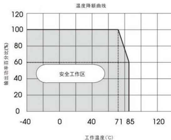
ULP20-H2424*温度降额曲线
