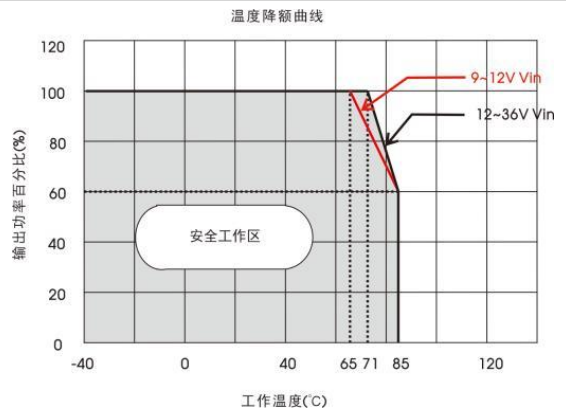
ULP20-H2412*、ULP20-H2415 温度降额曲线
