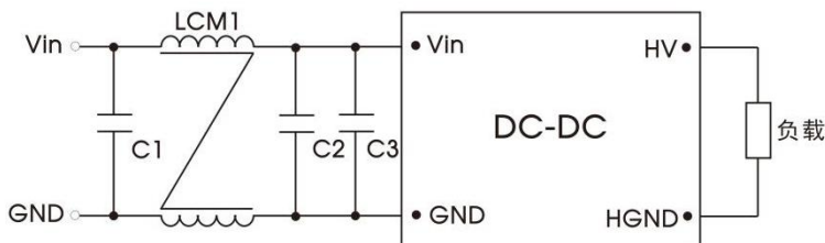
图 2 EMC 推荐电路
