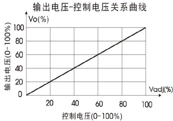
(注: 100% Vadj 等于 5.0VDC (Typ.)) 图 3 输出电压与控制电压关系曲线
