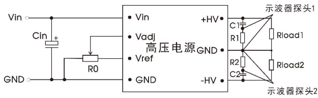
图 4 纹波噪声测试推荐电路
