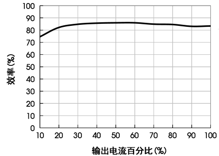
DS1-A0505 效率Vs输出负载 (Vin=5V)
