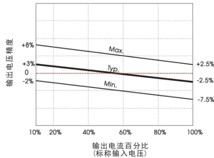
12/15/24VDC 输入其他输出 误差包络曲线图
