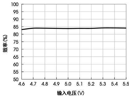
DS1-A0505 效率Vs输入电压 (满载)
