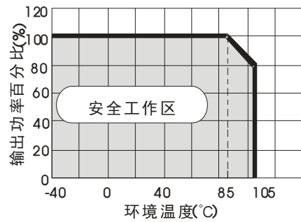
5VDC 输入 温度降额曲线图
