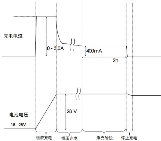
两节电池未联接中线串联充电模式
