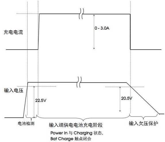
电池充电方式 电池充电模式
