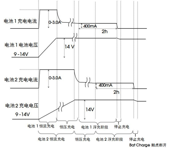
两节电池联接中线串联充电模式
