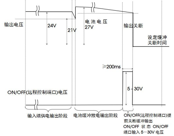
ON/OFF 状态定义
