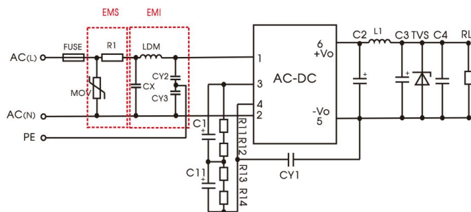
推荐电路 5
