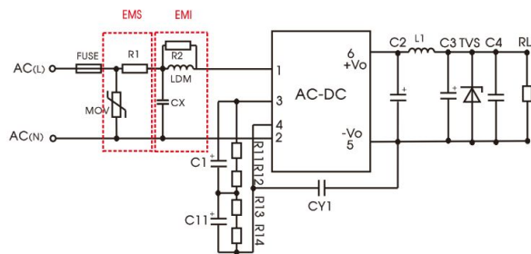
推荐电路 3
