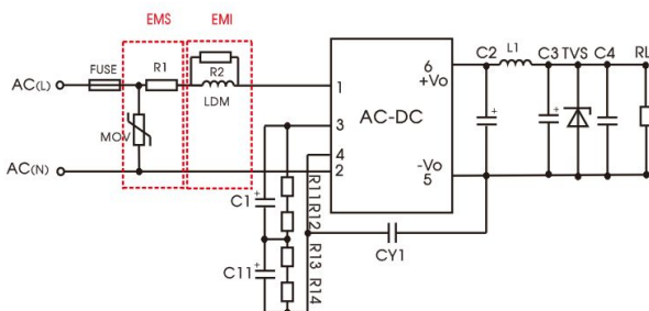
推荐电路 4
