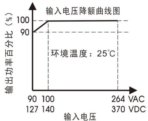
AOF350-Bxx-C 输入电压降额
