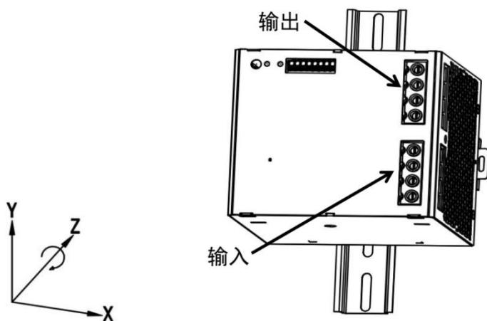
旋转安装位置 (270° Z-轴)
