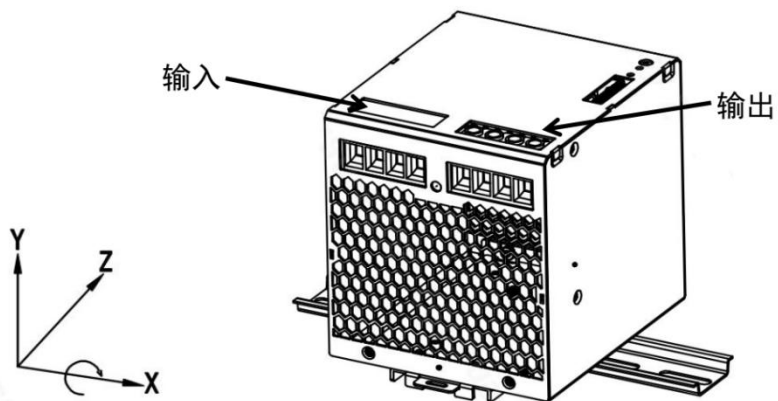
旋转安装位置 (90° X-轴)
