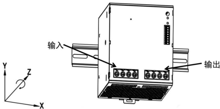
旋转安装位置 (0° Z-轴)
