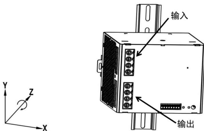
旋转安装位置 (90° Z-轴)
