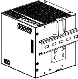
② 安装通用DIN导轨适配器 (侧面反装，需撕标签纸)
