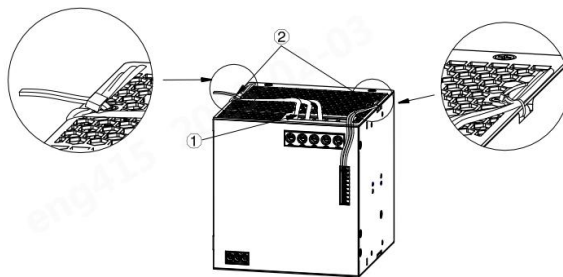
① 端子接上连接线后，铺设和对齐连接线； ② 通过外壳两侧的缺口，用电缆捆扎条，固定连接。
