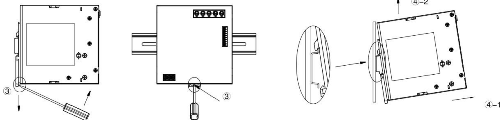
拆卸步骤③-④
