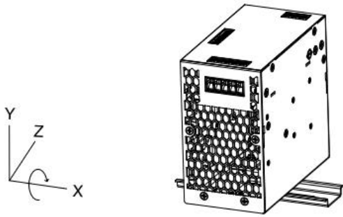
旋转安装位置(90° X-轴)
