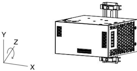
旋转安装位置(90° Z-轴)
