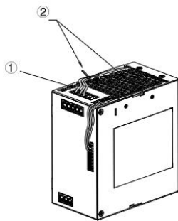
① 端子接上连接线后，铺设和对齐连接线； ② 通过外壳两侧的缺口，用电缆捆扎条，固定连接。
