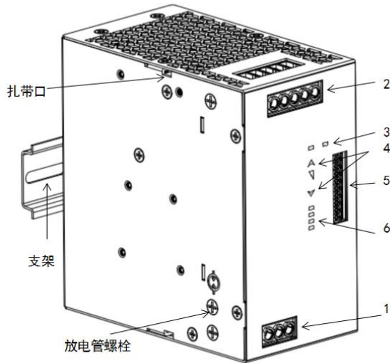
图 1: AIHF480-Bxx 外观信息
